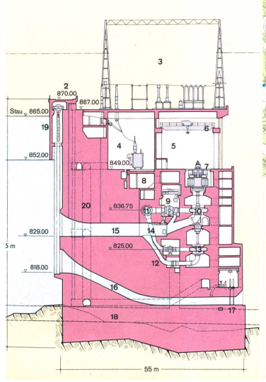
Querschnitt
