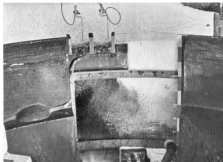
Bild 4 Blick von der Talseite durch die Plexiglasmodellstau-mauer. Es ist ersichtlich, wie das Lawinenmaterial während der Eintritts-phase teilweise bis gegen die Wasserfassung (unten rechts) und die Grundablässe (unten Mitte) hinuntertaucht. In den beiden Oeffnungen der Hochwasserentlastung sind die Widerstandsmesspegel sichtbar.
