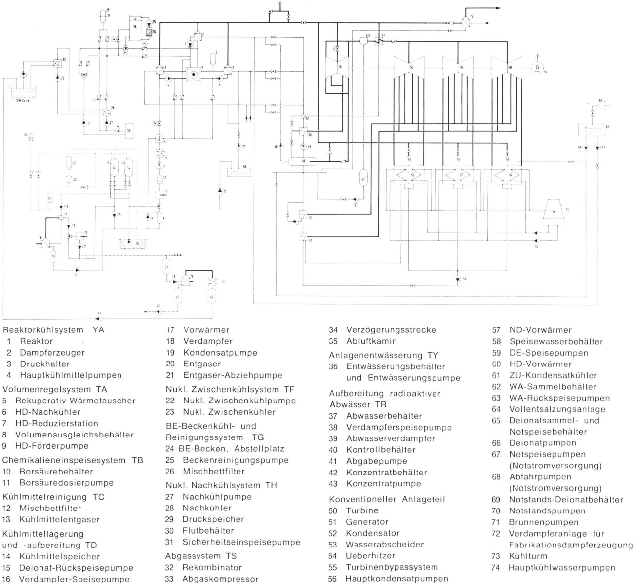
Bild 3 Vereinfachtes Uebersichts-Schaltbild des Kernkraftwerks Gösgen.
