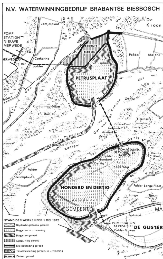
Bild 3 Uebersichtsplan der Speicherbecken im Brabanter Biesbosch, die die Rohwasserversorgung der Stadt Rotterdam und der Provinzen Brabant und Zeeland für die fernere Zukunft sicherstellen.
