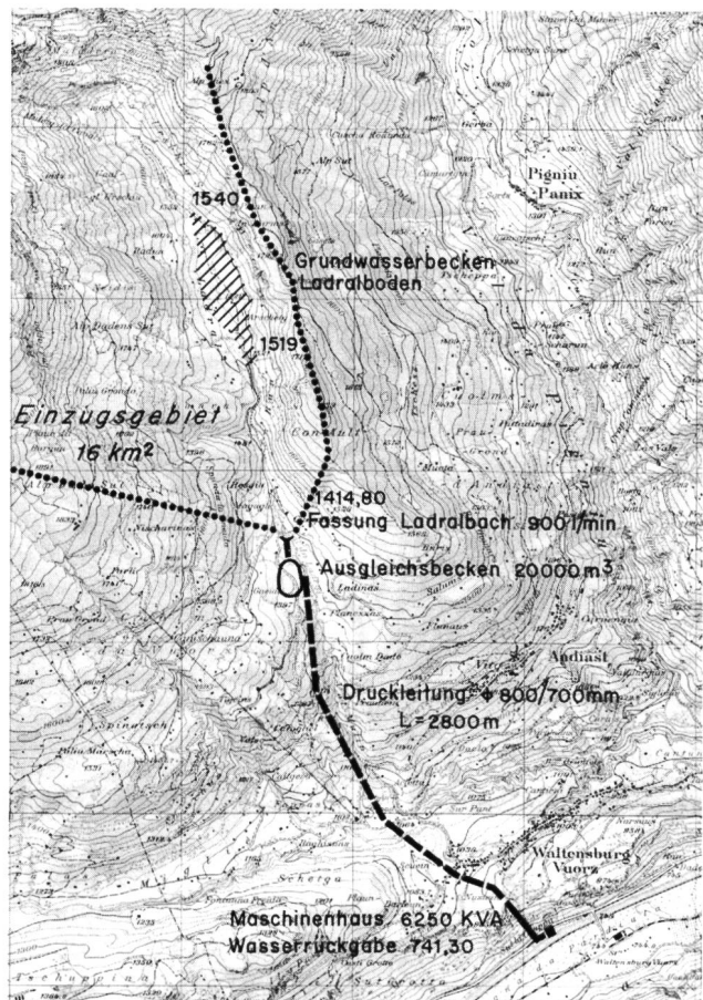
Bild 1 Uebersichtsplan über die Anlagen des neuen Kraftwerks Ladrall; Ausnützung des Ladrallbaches als Einstufenwerk mit Fassung auf Kote 1414,80. Ausschnitt aus der Schweizerischen Landeskarte 1:25 000, verkleinert auf 1:50 000, reproduziert mit Bewilligung der Eidg. Landestopographie vom 1. März 1976.
