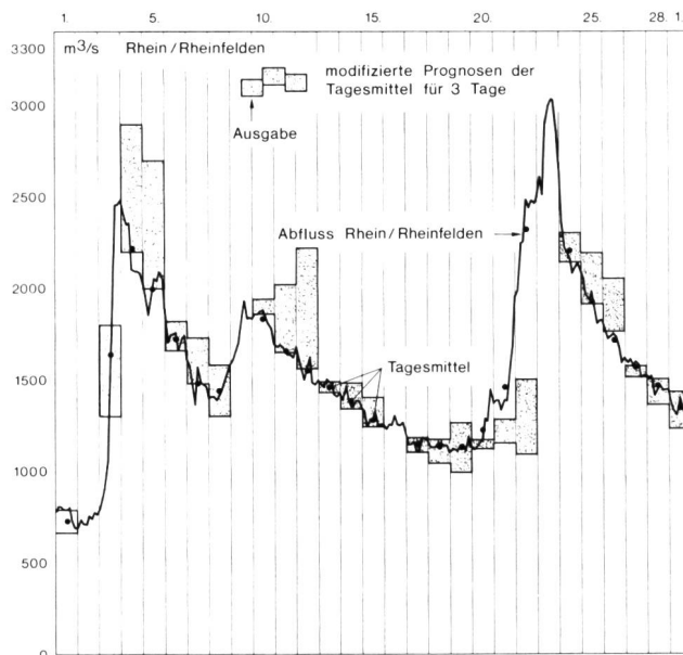
Bild 6 Rhein bei Rheinfelden. Kurzfristprognosen für den Abfluss. Vorhergesagte Tagesmittel des Ausgabetages und der beiden nächstfolgenden Tage (unterer Wert mit 90 %, oberer mit 10 % Überschreitungswahrscheinlichkeit), im Vergleich zu den beobachteten Werten. Abflussganglinie des Februars 1970.
