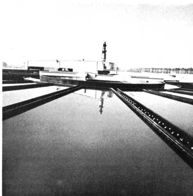
Bild 9. Flockungsreaktor der neuen Anlage. Décauteur flocculateur de la nouvelle station de traitement.
