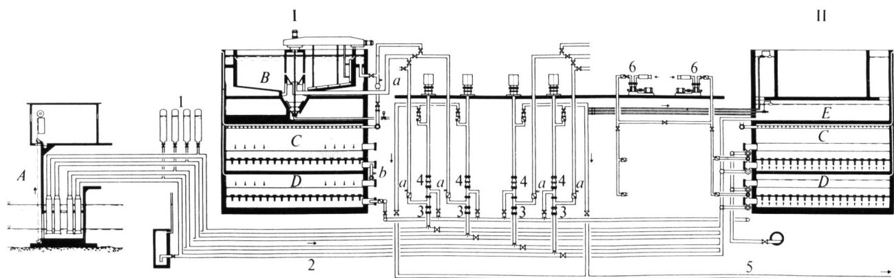
Bild 4 Schema der alten Aufbereitungsanlage. I Filtration, II Spülung; A Wasserfassung, B Grobteilabscheider, C Vorfilter, D Hauptfilter, E Spülwasserreservoir; 1 Vakuunkessel, 2 Saugleitungen, 3 Rohwasserpumpen, 4 Reinwasserpumpen, 5 Reinwasserleitung, 6 Spülluftgebläse; a Flockungsmittel, b Chlor.
