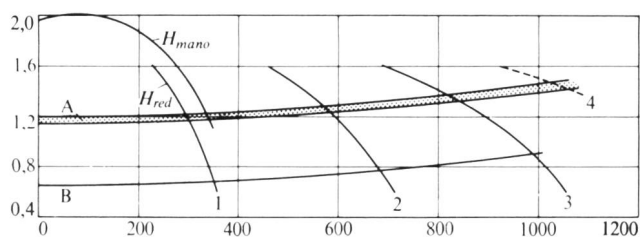
Bild 13. Pumpenkennlinien beim Einzelbetrieb der neuen Anlage. 1 bis 4 Kennlinien der Reinwasserpumpen (oben) und der Rohwasserpumpen (unten); H_{mano} Manometrische Förderhöhe, H_{red} Manometrische Förderhöhe bei Drosselung; A Zulässiger Druckbereich, B Kennlinie der Rohwasser-Saug- und -Druckleitungen.
