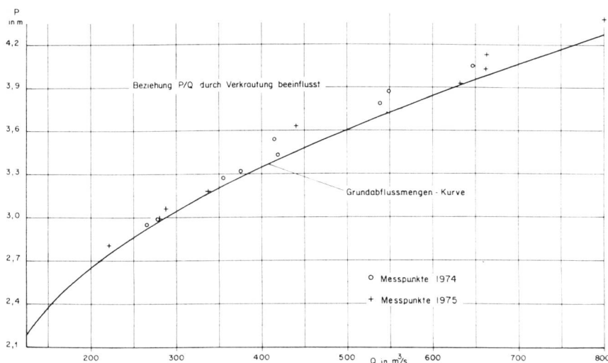
Bild 2. Messstation Rhein-Neuhausen. Abweichung (Streuung) der 9 bzw. 7 Eichmesswerte in den Jahren 1974 und 1975 von der früher gültigen P/Q -Beziehung zufolge Verkrautung. Das Ausmass der Abweichung kann als Pegelstand-Überhöhung (in cm) abgelesen werden.
