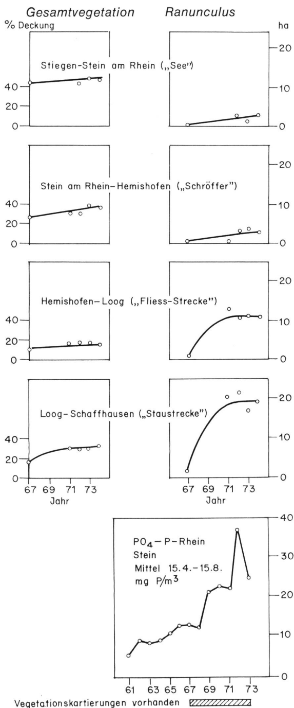
Bild 2. Die Makrophyten-Vegetation im Oberrhein. Nach Zahlen aus [3], J. Bühler, 1976. Links die Gesamtvegetation als prozentuale Dekung der Flusssohle; rechts die Bedeckung der Flusssohle durch Ranunculus fluitans in ha. Als Vergleich dazu wird unten die Zunahme der \text{PO}_4\text{-P} -Fracht im Rhein in \text{mg P/m}^3 gegeben. Die unterschiedliche Ausbreitung des Ranunculus zeigt seit 1971 wenig Veränderungen.
