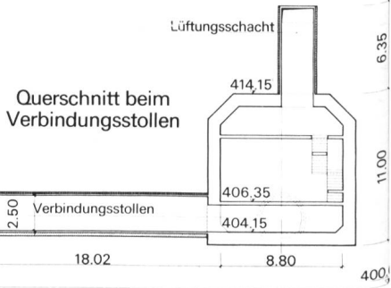
Bild 1. Grundriss und Querschnitt des Unterwerks Katz des Elektrizitätswerks der Stadt Zürich.
