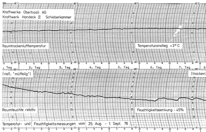
Bild 6. Absenkung der Luftfeuchte von 82 auf 40% relative Luftfeuchte in der Schieberkammer Handegg II, der Kraftwerke Oberhasli AG.
