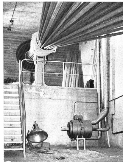
Bild 9, rechts. Blick in einen Kontrollraum der Trage-Seil-Widerlager einer Brücke über See mit Luftentfeuchter.
