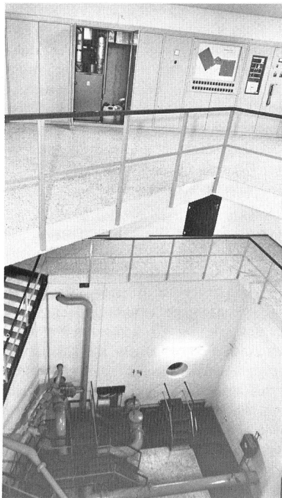
Bild 6. Absenkung der Luftfeuchte von 82 auf 40% relative Luftfeuchte in der Schieberkammer Handegg II, der Kraftwerke Oberhasli AG.
