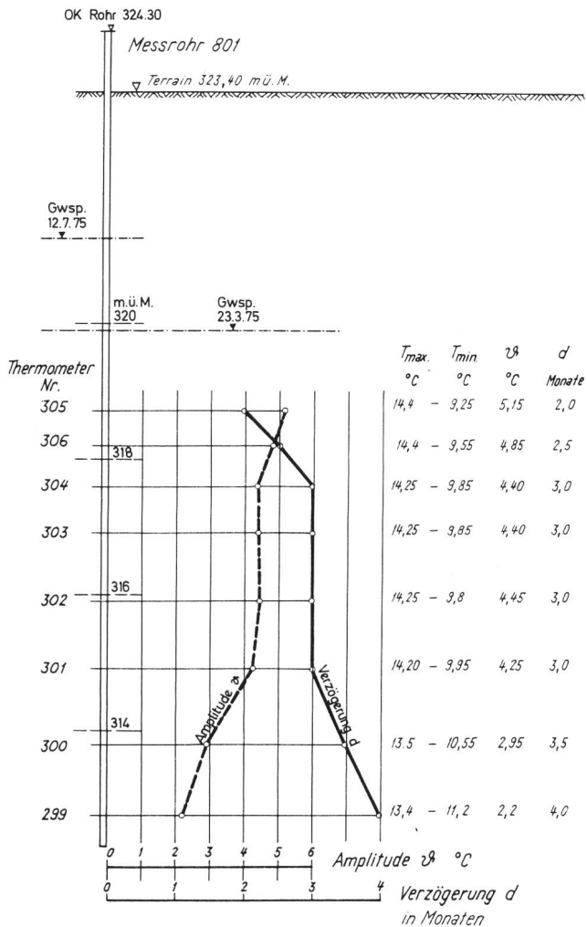
Bild 8. Amplitude \Delta 1975 und Verzögerung zur Aare d in Funktion der Tiefe unter Terrain bei «diffuser» Temperaturschichtung beim Rohr 801.
