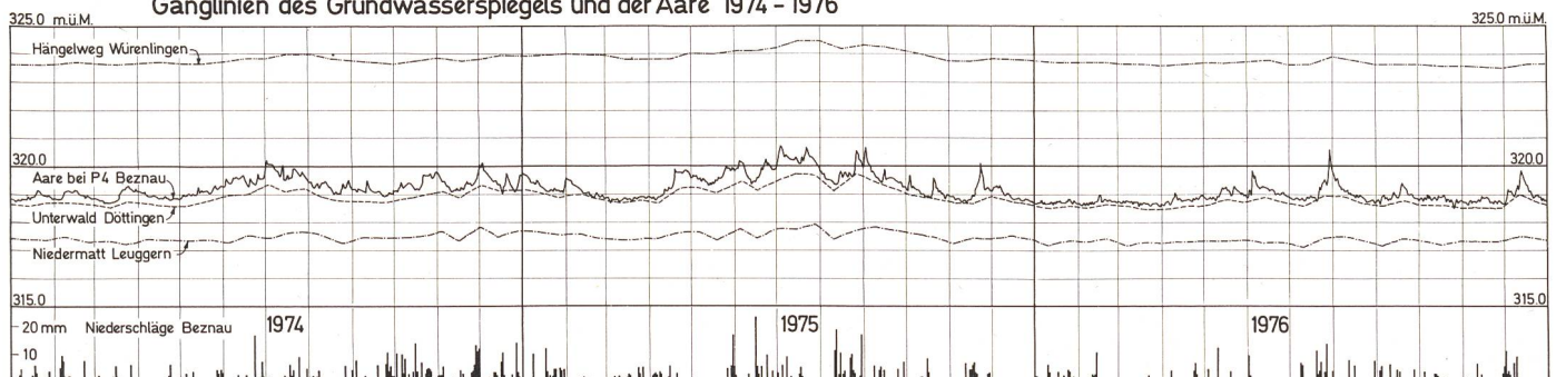
Ganglinien des Grundwasserspiegels und der Aare 1974 - 1976
