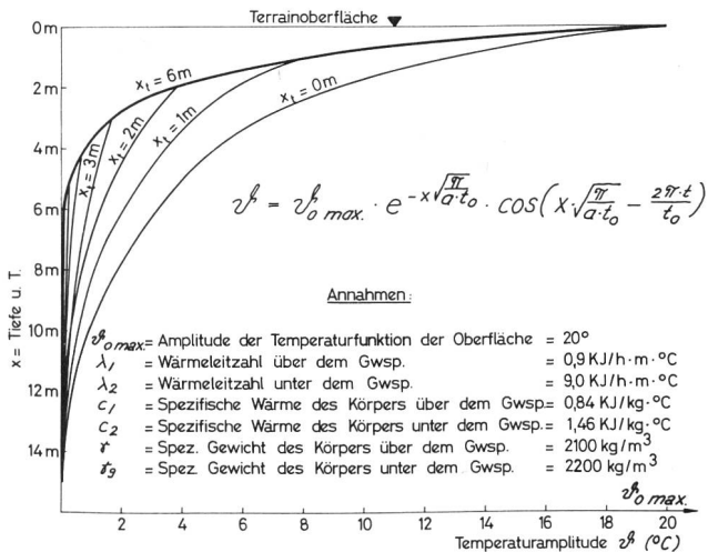
Bild 6. Dämpfung der Jahresamplitude \vartheta der Grundwassertemperatur in Funktion der Tiefe unter Terrain x für verschiedene Trockentiefen x_1 (nach E. Gröber 1955).
