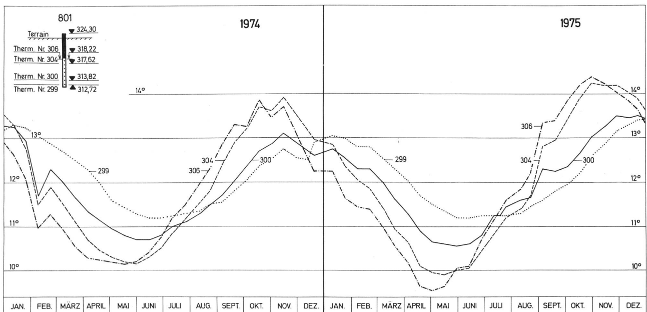
Bild 7. Ganglinien von 4 Thermometern am Rohr 801 auf der Bezau-Insel mit «diffuser» Temperaturschichtung.
