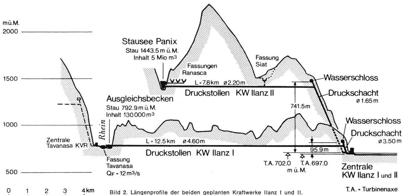
Bild 2. Längsprofile der beiden geplanten Kraftwerke Ilanz I und II.
