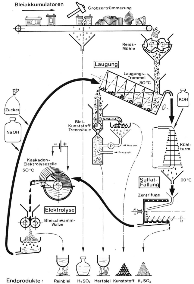
Bild 1. Bleirückgewinnung aus Akkumulatoren mit einem geschlossenen Kreisprozess und wiederverwendbaren Endprodukten. Abteilung für industrielle Forschung des Institutes für technische Physik der Eidg. Technischen Hochschule Zürich.
