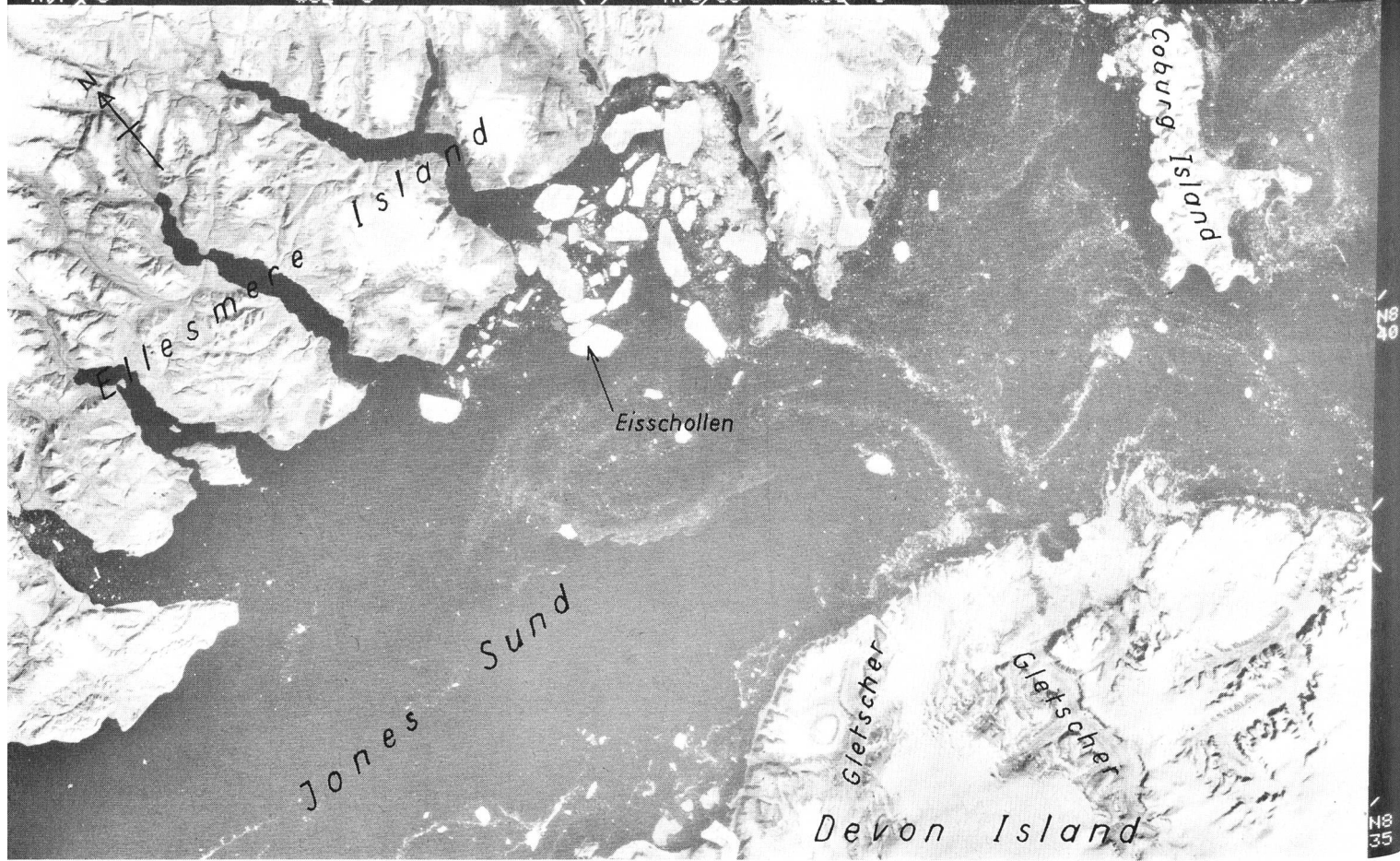
Bild 1. Satellitenaufnahme (LANDSAT) vom 5. August 1973. Im Masstab von etwa 1 : 950 000 sind Eisschollen im Jones Sund, Gletscher auf Devon Island sowie Coburg Island zu erkennen (kanadische Arktis).
