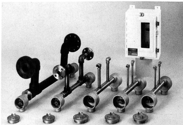
Bild 1. Mapco-Nusonics-Ultraschall-Durchflussmesser.
