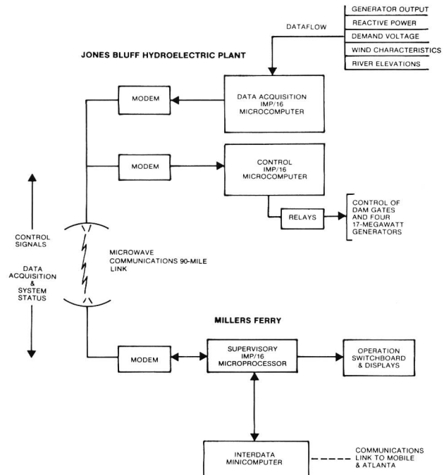
Bild 2. Das Blockdiagramm zeigt die Verbindungen zwischen den Mikrocomputern und den Minicomputern für die Steuerung und Überwachung der Wasserkraftanlage Jones Bluff von Millers Ferry aus.
