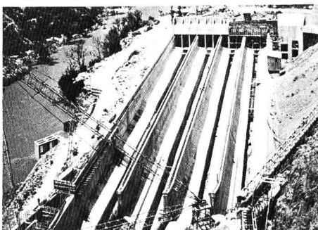
Sandabzugsvorrichtung BIERI im Rio Mantaro, Peru
