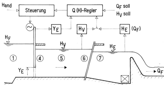
Bild 3. Automatisierung des Wasserhaushaltes.
