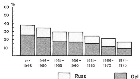
Bild 8. Die Altersverteilung der Heizkessel und die je dazugehörigen Beanstandungen in %.
