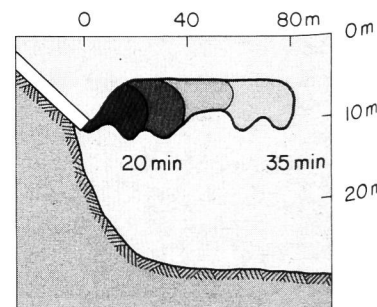
Bild 16. Zeitlicher Verlauf einer Abwassereinleitung in den Vierwaldstättersee vom 28. August 1973 (nach Ambühl).
