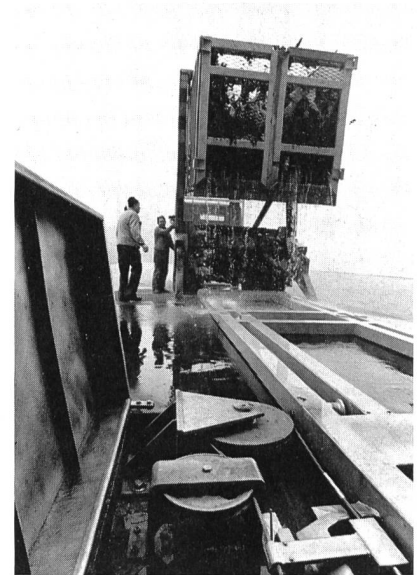
Bild 1, links. Das am Maschinenhausrechen mit der Rechenreinigungsmaschine dem Wasser entnommene Geschwemmelmateriale (Äste, Laub, Moos, Seegras, Autopneus usw.) wird über eine Einlaufrinne in den im Geschwemmelsraum bereitstehenden Grosscontainer mit 24 m 3 Fassungsvermögen gespült.
