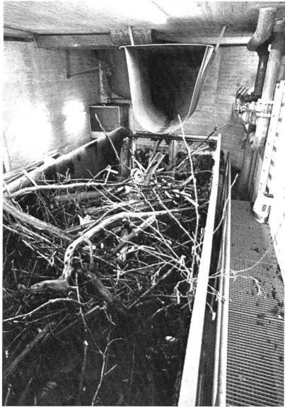
Bild 1, links. Das am Maschinenhausrechen mit der Rechenreinigungsmaschine dem Wasser entnommene Geschwemmelmateriale (Äste, Laub, Moos, Seegras, Autopneus usw.) wird über eine Einlaufrinne in den im Geschwemmelsraum bereitstehenden Grosscontainer mit 24 m 3 Fassungsvermögen gespült.
