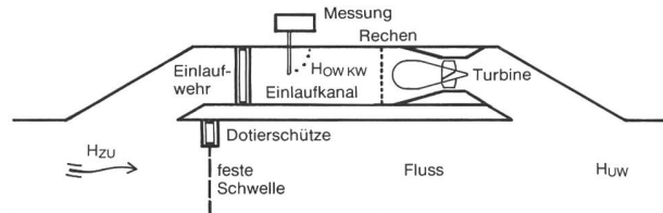
Bild 1a. Laufwasserkraftwerk mit Einlaufwehr.
