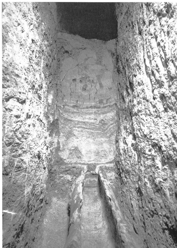
Bild 8. Eupalinostunnel, Samos. Rohrgraben mit aufgeschlagener Tonrohrleitung, Sinterablagerungen und Bodeneinschwemmungen.
