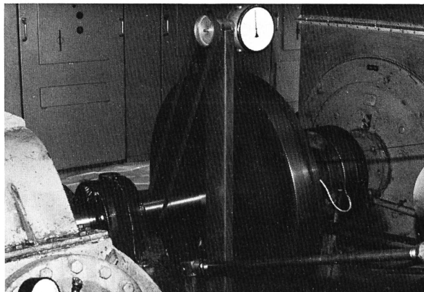
Bild 4. Zustand alt, mittleres Stützlager, Schwungrad und flexible Kupplung.
