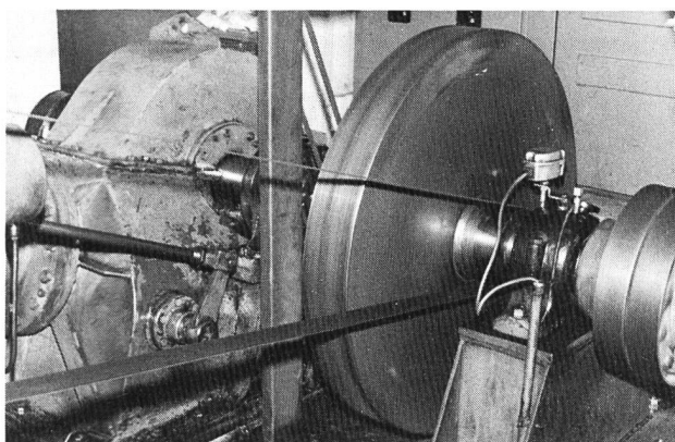
Bild 1. Zustand alt, Turbinengehäuse und Schwungrad.
