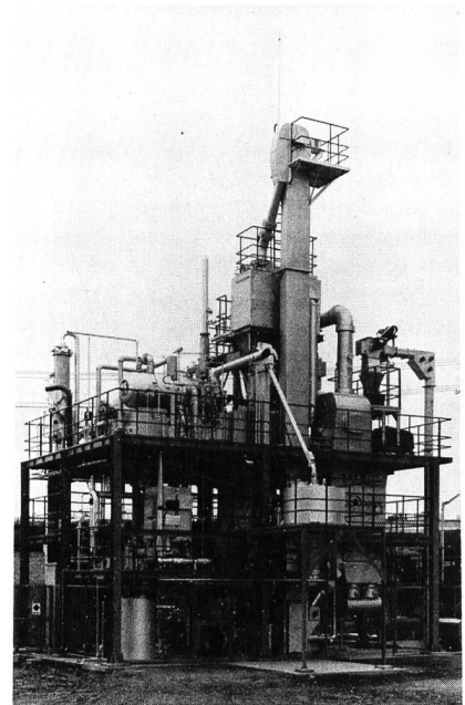
Klärschlamm-Verbrennungsanlage in Kyoto/Japan.
