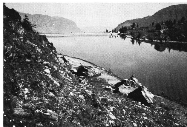
Bild 3. Bereits schmale Bermen vermögen rollende Blöcke abzufangen (Süd- ufer Bannalpsee).
