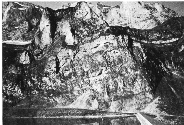
Bild 2. Felssturzgefahr oberhalb des Bannalp-Dammes, Übersicht. Als Schutz wurde über dem bestehenden Damm eine ca. 3 m dicke Schutzschicht aus Gehängeschuttmaterial geschüttet.
