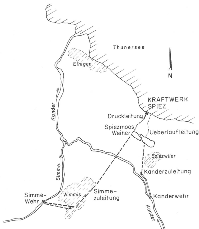
Bild 1. Übersichtsskizze Kraftwerk Spiez im Maßstab von etwa 1:60.000.
