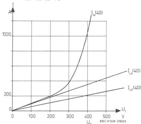
Bild 8. Leerlaufcharakteristik Asynchronengenerator, pQO 500 ab 6 bei 40 Hz.
