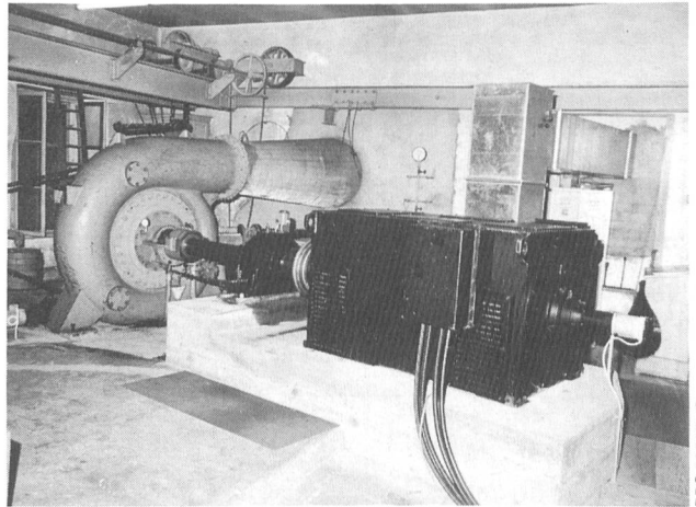
Bild 10. Wasserkraftwerk Moutier. Links die Francisturbine, welche den rechtsstehenden Asynchronengenerator pQO 500 ab 6 in der Bauform IM B3 antreibt. Schutzart IP 23. Daten des Generators: U_n = 400 \text{ V} , f_n = 50 \text{ Hz} , n_n = 1008 \text{ min}^{-1} , P_n = 900 \text{ kW} , \cos \phi_n = 0,85 , Durchgangsdrehzahl = 2000 \text{ min}^{-1} . Hinter dem Generator befindet sich der Abluftkanal. Die Warmluft heizt mittels Wärmeaustauscher eine Dienstwohnung im selben Gebäude (Verlustleistung 10...30 kW bei \frac{1}{4} \dots \frac{4}{4} -Last). Inbetriebnahme: 1979.
