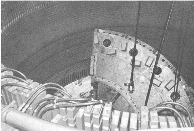
Bilder 5 und 6. Da eine Zwischenwelle fehlt, muss nicht nur die Pump- turbine selbst, sondern auch der Motorgenerator demontiert werden. Die Satorbohrung ist nicht gross genug, um den Ausbau des Turbinendeckels im ganzen zu ermöglichen – eine weitere Komplikation. Hier (Bild 5)
