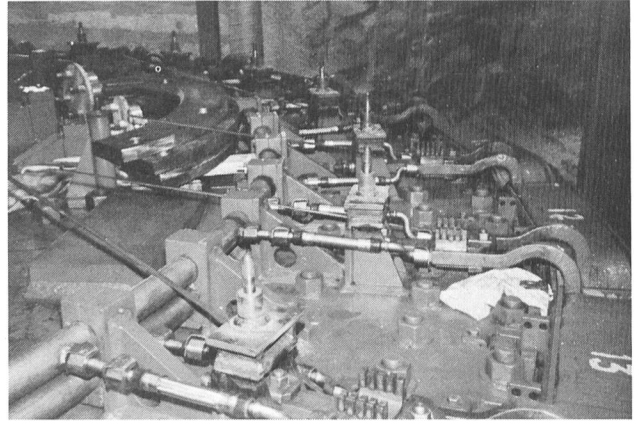
wird gerade eine Hälfte des Turbinendeckels hochgezogen. Im Vordergrund erkennt man Schlauchverbindungen und Zuführungsrohre zur wassergekühlten Satorwicklung. Vibrationen verursachen hier häufig Störungen, ebenso an der direkt wassergekühlten Rotorwicklung (Bild 6).
