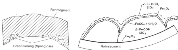
Bild 11. Schnittzeichnung der Rostablagerung.
