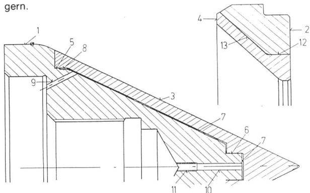
Düsennadel und Düsennadelring zu einer Peltonturbine. 1 Düsennadel-Körper, 2 Düsennadel-Kappe, 3 Düsennadel-Einsatz, 4 Zentrier-Sitz, 5 Zentrier-Sitz, 6 Klebefuge, 7 Gewinde, 8 Klebstoff-Entlastungsbohrung, 9 Klebstoff-Entlastungsbohrung, 10 Abpress-Gewinde, 11 Press-Sitz, 12 Klebefuge, 13 Klebefuge.
