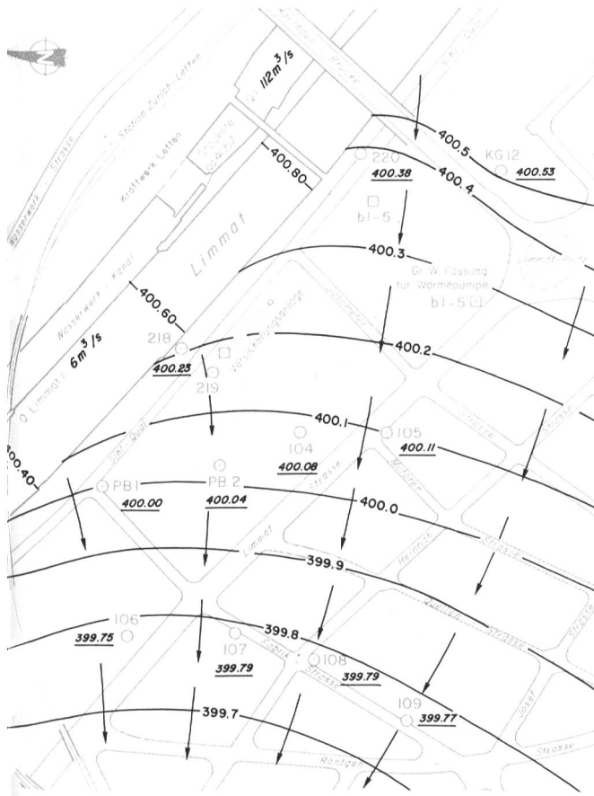
Bild 4. Isohypsen des Grundwasserspiegels am 1. Juni 1983 bei Ruhelage (hoher Mittelwasserstand). Massstab 1:5000.
