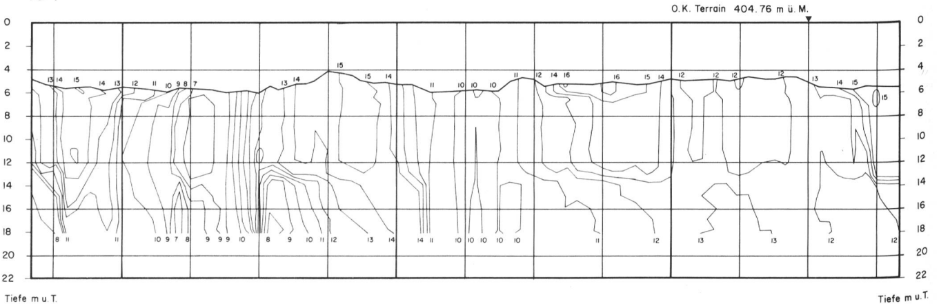
Bild 9. Isoplethen der Grundwassertemperatur bei den Messstellen PB 2 und IO4.
