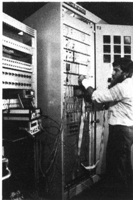
Elektronischer Turbinenregler, wie er auch im grössten Pelton-turbinen-Kraftwerk der Welt eingesetzt wird.
