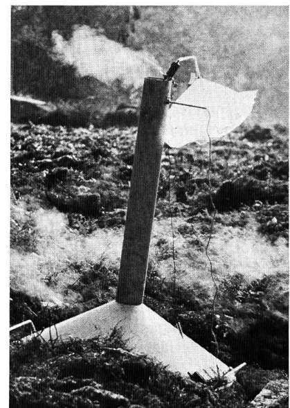
Bild 6. Biofilter aus Fastertorf und Heidekraut zur Reinigung der Abluft aus der Schlamm-trocknungs-anlage. Entnahme der Geruchsproben über einem Trichter von 1 m 2 Grundfläche.
