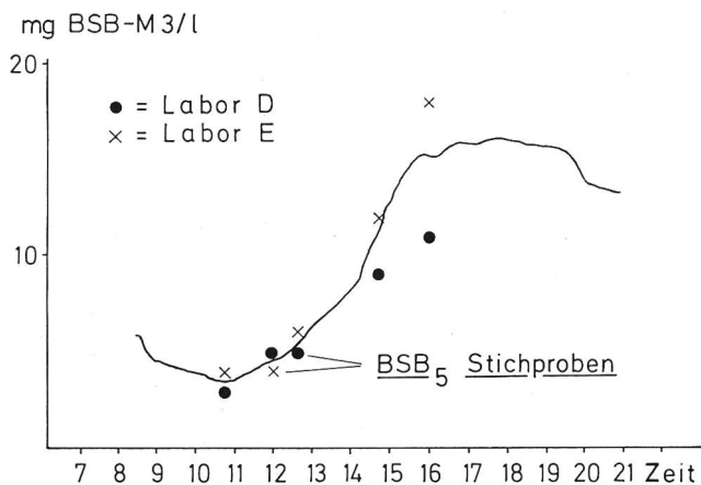
Bild 5. Eichtung des BSB-M3 auf den BSB 5 am Auslauf der Nachklärung.
