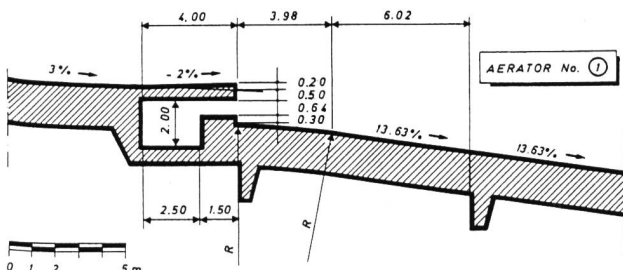
Bild 8. Details eines Sohlenbelüfters, Mosul Damm, Schussrinne.
