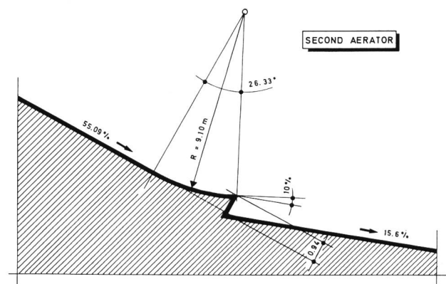
Bild 9. Sonderausführung eines Belüfters an einem einspringenden Knick im Längenprofil der Schussrinne. Aghios Nikolaos Schussrinne.
