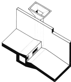
Bild 5. Bauformen von Belüftern.
