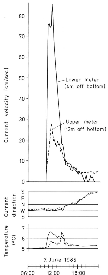
Bild 13. Aufzeichnung eines zuflussbedingten Dichtestroms im Rhonedelta des Genfersees infolge des Hochwassers vom 7. Juni 1985 ( 620 \text{ m}^3/\text{s} ). Messposition: 5 km westlich der Rhonemündung in 200 m Tiefe. Der Dichtestrom zeichnet sich zwischen 10.30 und 16.00 Uhr durch hohe Strömungsgeschwindigkeiten und erhöhte Temperatur aus.
