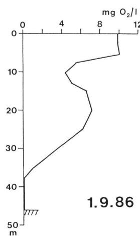
Bild 7. Typische Sauerstoffprofile im Hallwilsee vor und nach Beginn der see-internen Massnahmen (1. Zwangszirkulation, Dezember 1985 bis Mai 1986, Testbetrieb Tiefenwasserbelüftung, September 1986 bis November 1986, 2. Zwangszirkulation, November 1986 bis Mai 1987).
