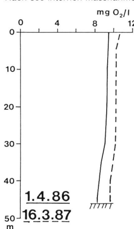
Bild 7. Typische Sauerstoffprofile im Hallwilsee vor und nach Beginn der see-internen Massnahmen (1. Zwangszirkulation, Dezember 1985 bis Mai 1986, Testbetrieb Tiefenwasserbelüftung, September 1986 bis November 1986, 2. Zwangszirkulation, November 1986 bis Mai 1987).
