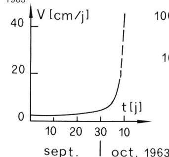
Figure 2. Evolution de la vitesse pour le glissement de Vajont en 1963.
