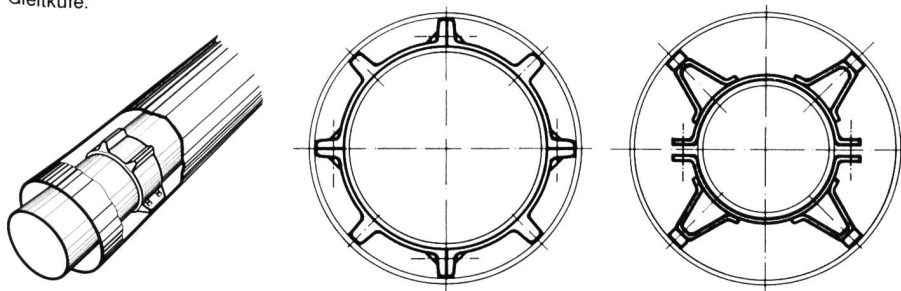
Bild 1. Mediumrohr/Mantelrohr/Gleitkufe.
