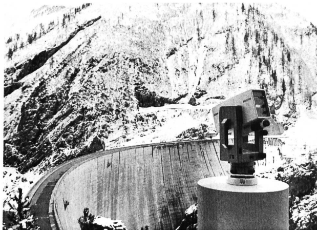
Das Mekometer Kern ME 5000: haargenauer Präzisionsdistanzmesser im wahrsten Sinne des Wortes!
