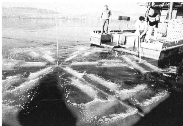
Bild 3b. Diffusor im feinblasigen Testbetrieb (Sommer).
