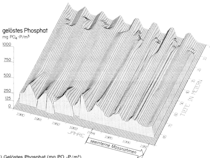
Bild 14. Saisonaler Verlauf der Phosphorkonzentrationen in der Seemitte vor und nach internen Massnahmen.
