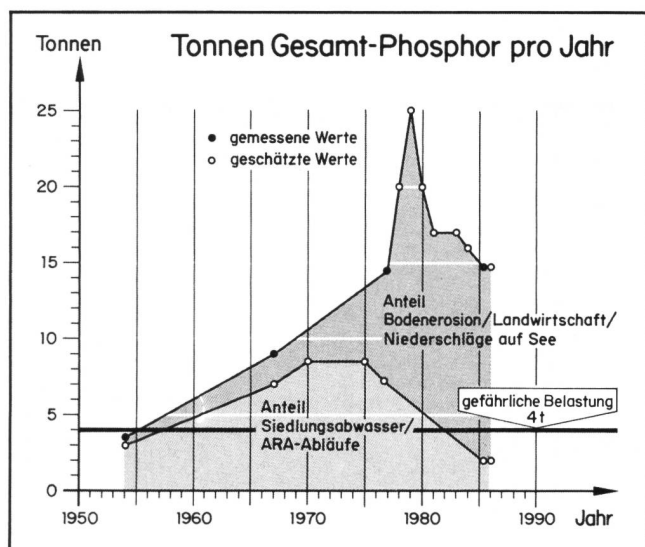
Bild 19. Jährliche Phosphorfrachten in Tonnen pro Jahr zum Sempachersee mit Anteil Siedlungsabwasser/Kläranlagen und Anteil Bodenerosion/Landwirtschaft/Niederschläge. Zuflussuntersuchungen 1954, 1966/67, 1976/77 und 1984/86.
