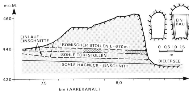
Bild 11. Zehnfach überhöhter Längsschnitt und Querschnitte in Sandstein (links) und Mergel (rechts) des Entwässerungstollens bei Hag-neck/BE.
