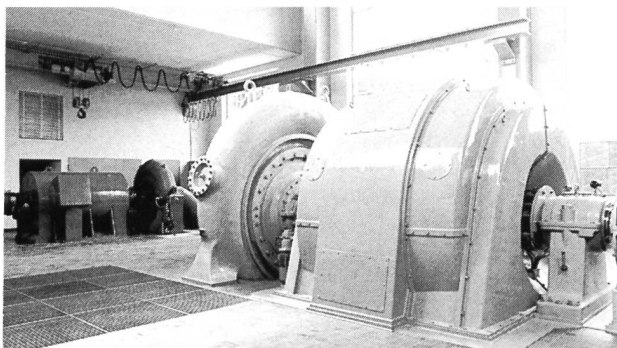
Bild 2. Kraftwerk Dallenwil. Rechts vorne eine der beiden Maschinengruppen von je 7500 kW Leistung, hinten links die neue Dotiermaschinengruppe mit einer Leistung von 2430 kW.
