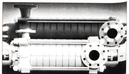
Identische Betriebspunkte werden mit einer reduzierten Stufenzahl und einer Steigerung des Wirkungsgrades erreicht.
