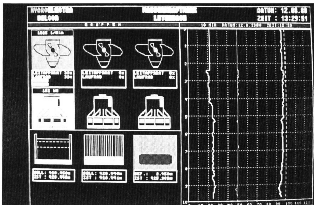
Bild 8. Hauptprozessbild des Helcon-Leitsystems. Alle übrigen Werte und Zustände können auf Knopfdruck angezeigt werden. Die Kurven rechts im Bild zeigen den Verlauf von Wasserstand, Leistung und Gefälle. Die Kurven können auch jederzeit für vergangene Stunden, Tage und Wochen (jeweils auf einer Seite) abgefragt werden. Dieselben Prozessdaten können auch via Fernbedienung überwacht werden.
