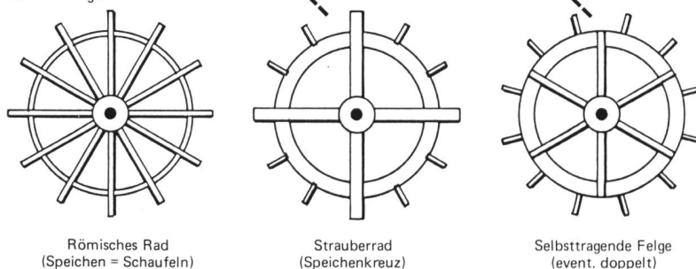
Bild 2. Typologie der Wasserräder.
