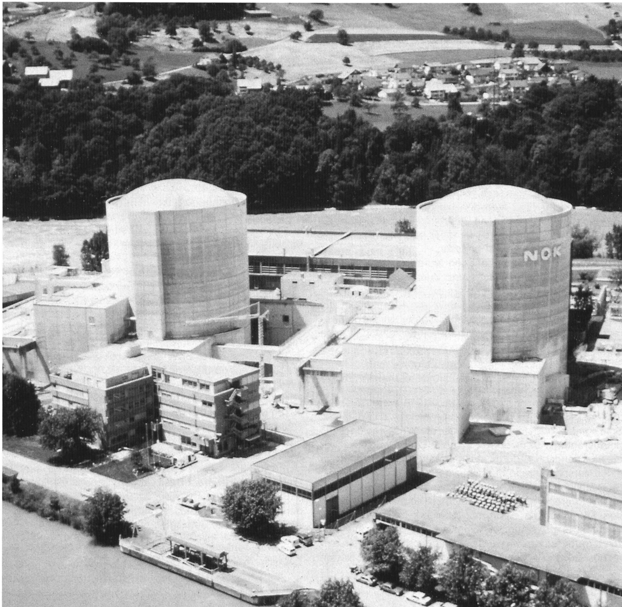
Bild 4. Im Jahre 1969 nahm Beznau I als erstes auf rein kommerzieller Basis erstelltes Kernkraftwerk der Schweiz den Betrieb auf. Bereits zwei Jahre später lieferte auch Beznau II Strom ans Netz. Die Leistung von Beznau I und II beträgt je 350 MW.
