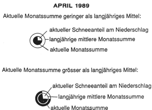
Bild 1. Aktuelle Monatssummen und Schneeanteile (berechnet) des Niederschlags an den Stationen des automatischen Netzes der SMA, verglichen mit den langjährigen mittleren Monatssummen für die beiden extremsten Monate des Winters 1988/89: Januar als sehr trockener Monat und April als sehr niederschlagsreicher Monat.
