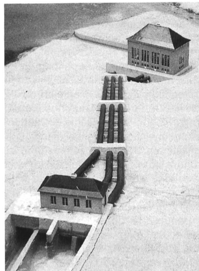
Bild 1, links. Das Wasserbaumodell 1:50 an der Landesausstellung 1939. Links ein Hochdruckspeicherwerk, in der Mitte ein Mitteldrucklaufwerk, rechts zwei geschleibeführende Wildbäche, die im See ein Delta bilden (Foto VAW).
