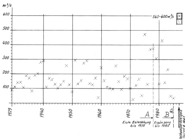
Bild 7. Hochwasserspitzen der Rovana bei Linescio in der Zeitspanne 1929–1985. A = Erste Berechnung bis 1978, B = Ergänzung bis 1985.
