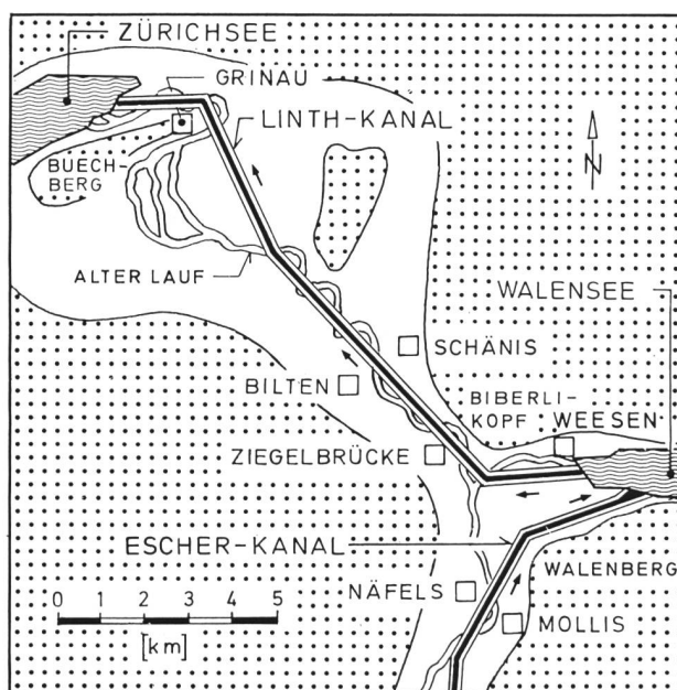
Bild 1. Links die einstige Situation des Bödels mit der vermeintlichen Lütshinenumleitung und der im 19. Jahrhundert durchgeführten Aarekorrektur; rechts die Situation der Linthebene mit der 1807–1816 durchgeführten Linthkorrektur zum Vergleich.
