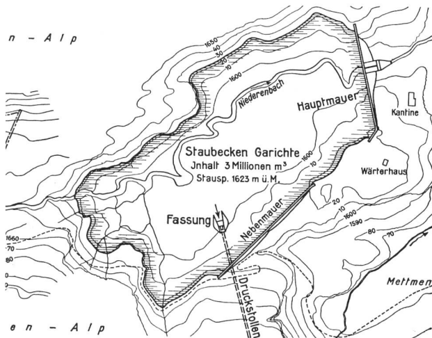
Bild 3. Situation des Stau Becken Garichte der Kraftwerke Sernf-Niedererbach AG. Aus «Schweizerische Bauzeitung» Band 106, 24. August 1935, S. 85.
