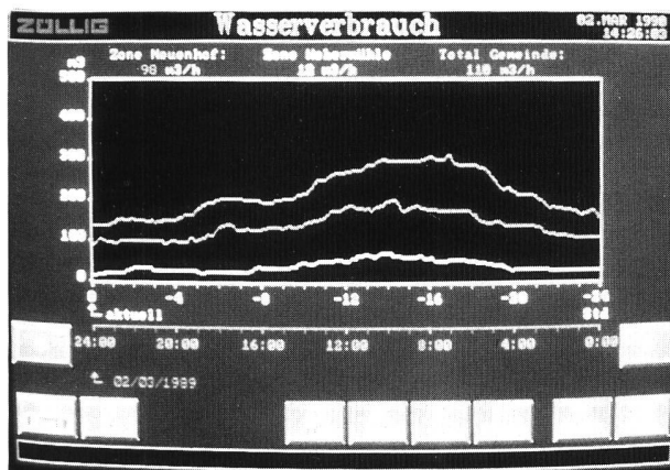
Bild 7. 24-Stunden-Programmsteuerung. Der Füllstand des Reservoirs «Rehweg» kann mit einer Sollwertkurve über den Tag (24 Stunden) vorgeplant werden. Dies kann zur Einsparung von Energiekosten (Pumpen) und zur optimalen Anpassung an den Bedarf interessant sein.
